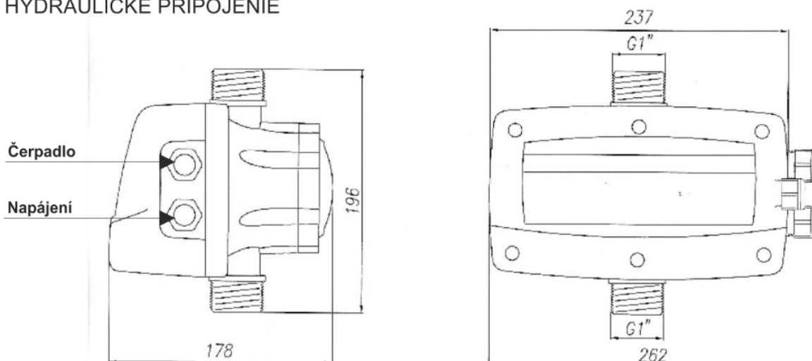
OBR 2: HYDRAULICKÉ PŘIPOJENÍ HYDRAULICKE PRIPOJENIE
