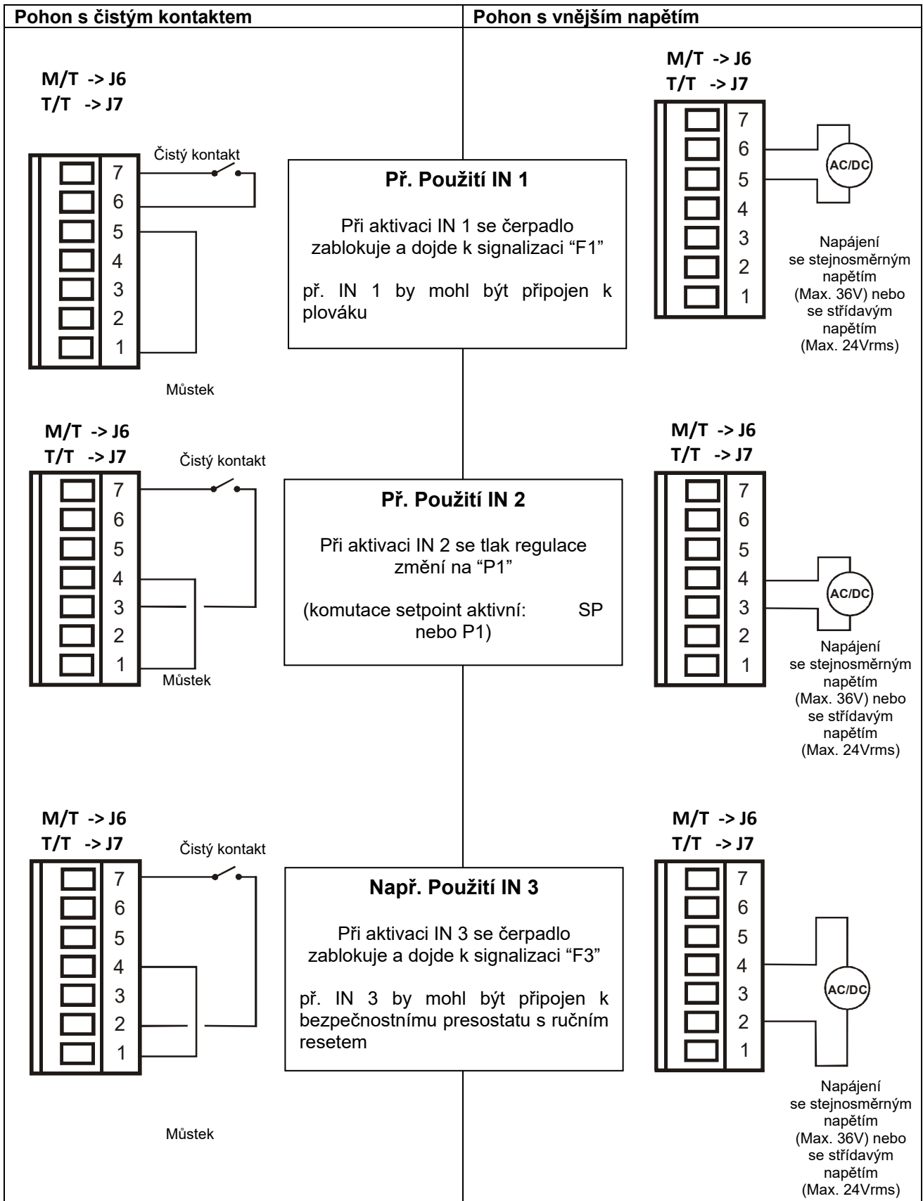
Obr. 2: Připojení vstupů
