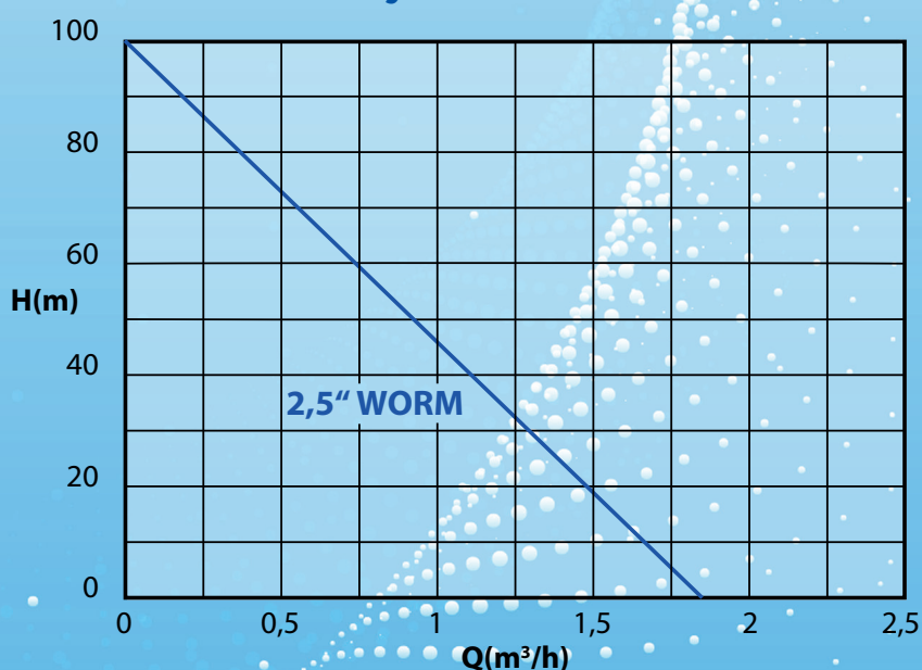
Výkonová křivka
